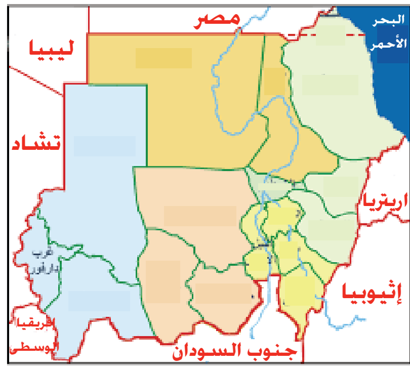
شكل ٢٩/٣: السودان وجيرانه.
