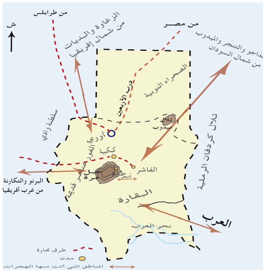
شکل ۱/۱۵: اقلیم دارفور
